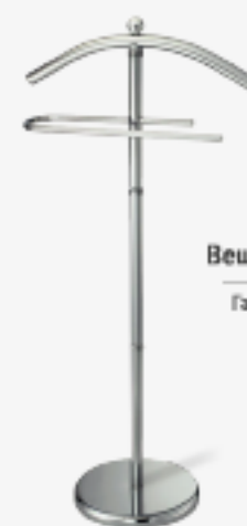
Вешалка CH-4043 Габаритные размеры: 280x460x1110 Материал: металл, дерево
