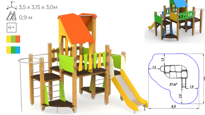
Детский игровой комплекс 311.53 Aviator 311.53
