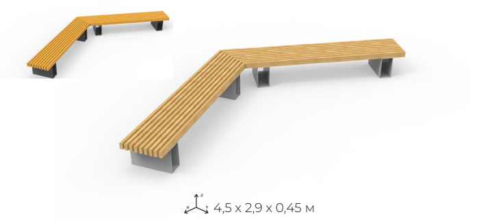
Скамейка «Бремен» Aviator 123.15.01
